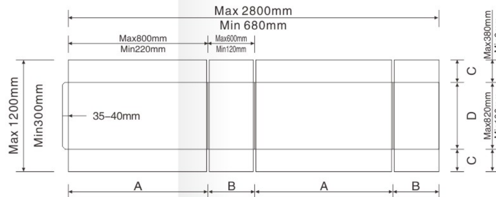
AXD-025 纸箱尺寸示意图，其他尺寸可定制
