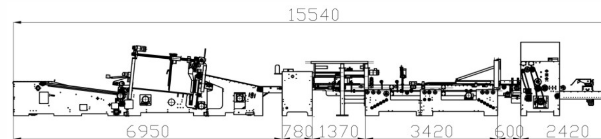
收纸部C 收纸部B 收纸部A 钉箱部 整形部 折纸部 送纸部
