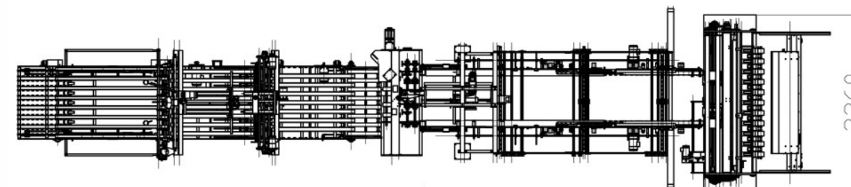
收纸部C 收纸部B 收纸部A 钉箱部 整形部 折纸部 送纸部
